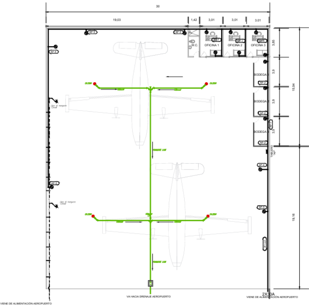
Propuesta de Hangar Lote 30x35
